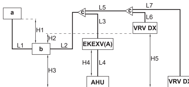
a Lämmönvaihdivyksikkö
