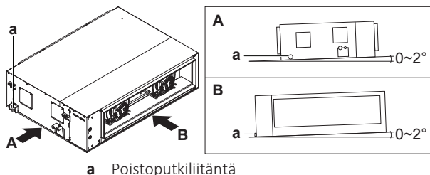
a Poistoputkiliitäntä
