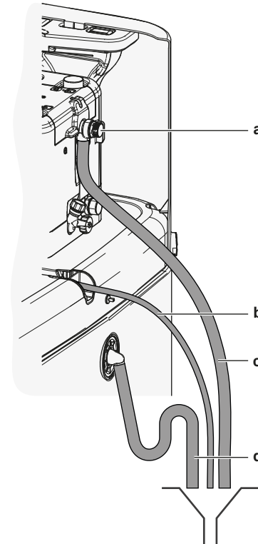
a Paineenalennusventtiili b Tippavesialtaan letku (toimitetaan lisävarusteena) c Paineenalennusventtiiliin tyhjennysletku (erikseen hankittava) d Varaajan tyhjennysletku (erikseen hankittava)
