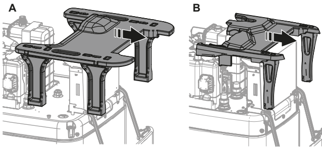
A Mallit, joissa on 500 litran varaajan säiliö B Mallit, joissa on 300 litran varaajan säiliö
