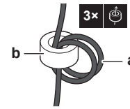
a Yhteiskytkenäkaapeli b Ferriittisydän
