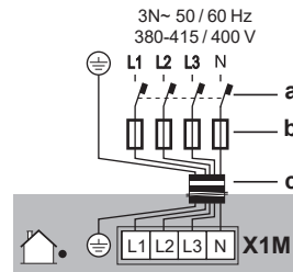
a Maavuosuosuokatkaisin b Sulake c Virransyöttökaapeli
