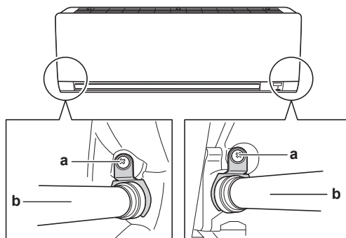
a Eristeen kiinnitysruuvi b Tyhjennysletku
